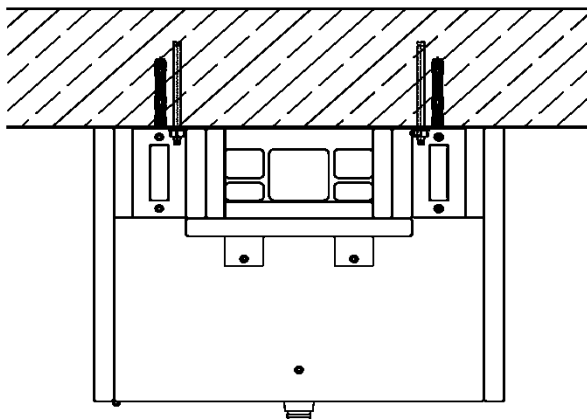
Draufsicht
