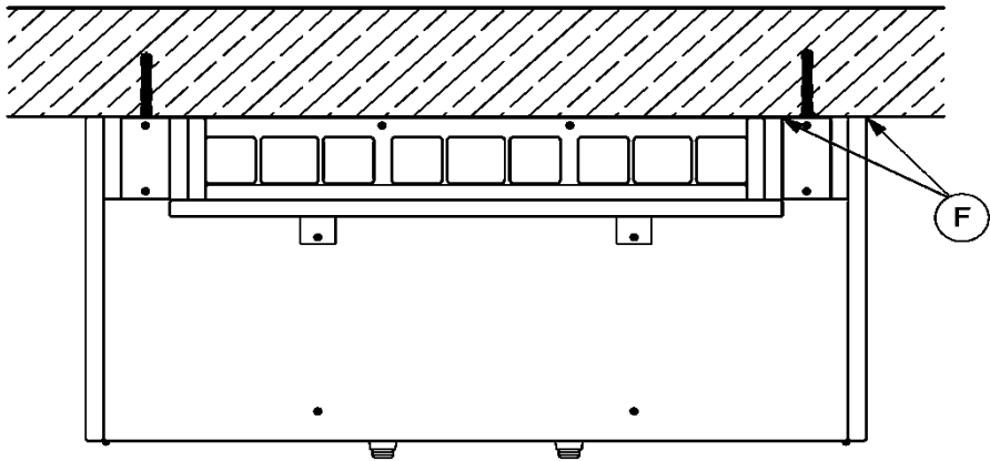
Untersicht
