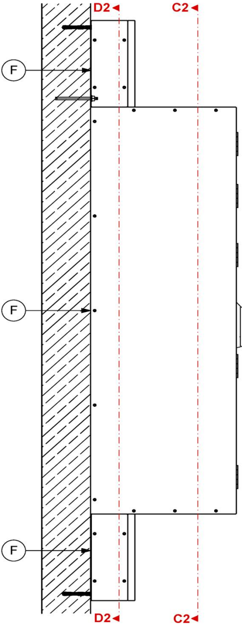
Seitenansicht
