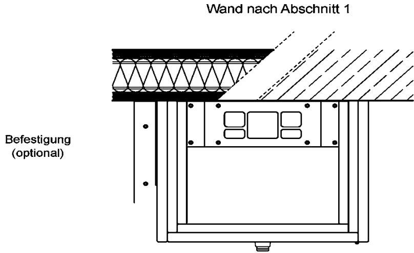
Untersicht
